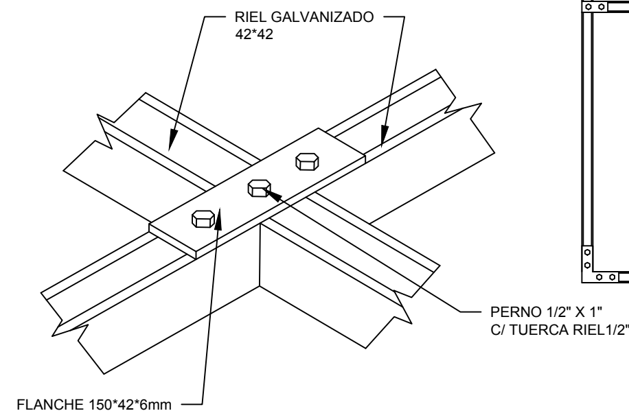
DET. ISOM. UNIÓN DE RIEL ESC. 1:4
