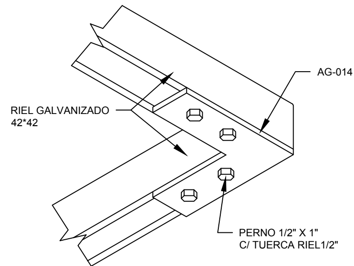
DET. ISOM. UNIÓN DE RIEL ESC. 1:4
