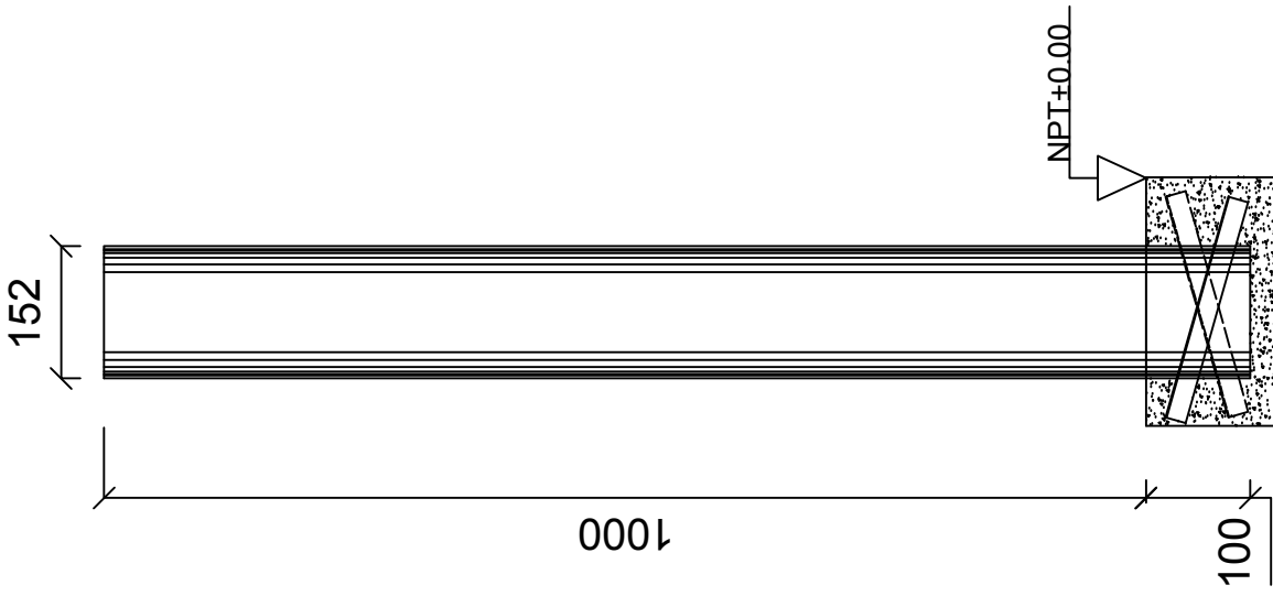
ELEVACIÓN FRONTAL ESC. 1:8
