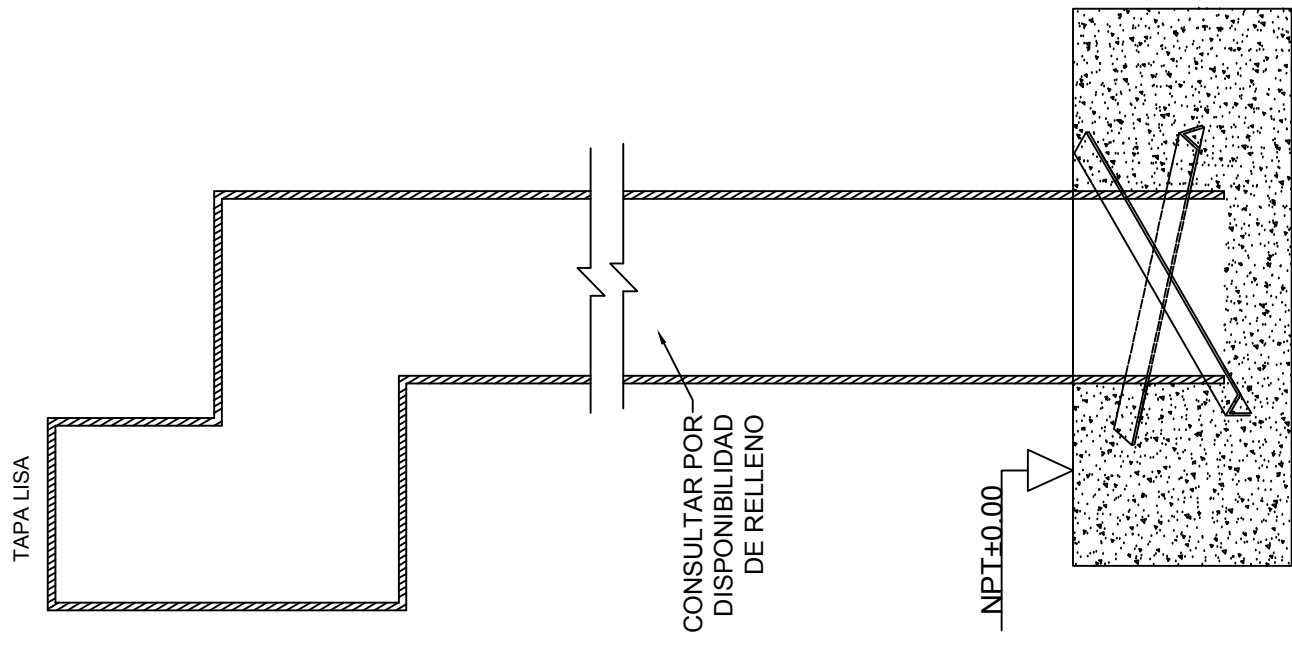
CORTE A-A ESC. 1:5
