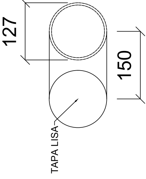
PLANTA ESC. 1:5
